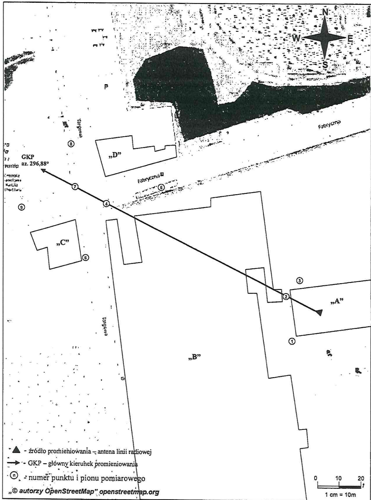
Rys. 1. Usytuowanie punktów i pionów pomiarowych w otoczeniu instalacji radiokomunikacyjnej Stacja Netia LODZB974-LODZM00449 Łódź, ul. Ks. Biskupa Wincenta Tymienieckiego 22/24
